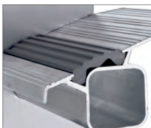
Lépcső ZARGES Safer Step technológiával
