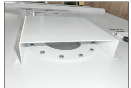
Biztonsági elem hasadó tárcsa: Védelem a hirtelen bekövetkező nyomásesésnél a környezetben
